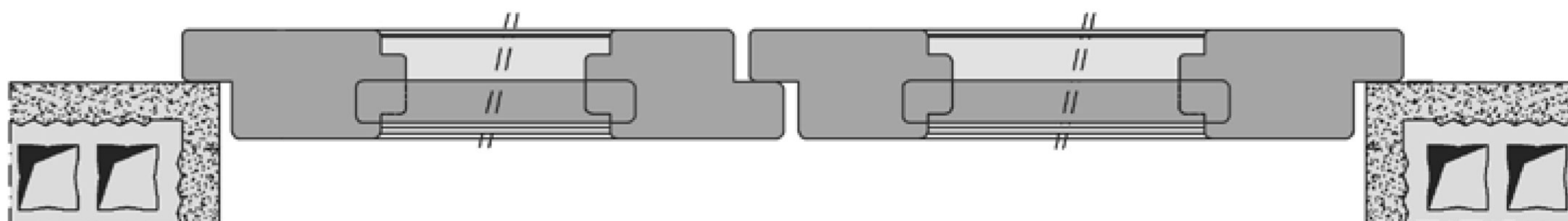
SEZIONE ORIZZONTALE
