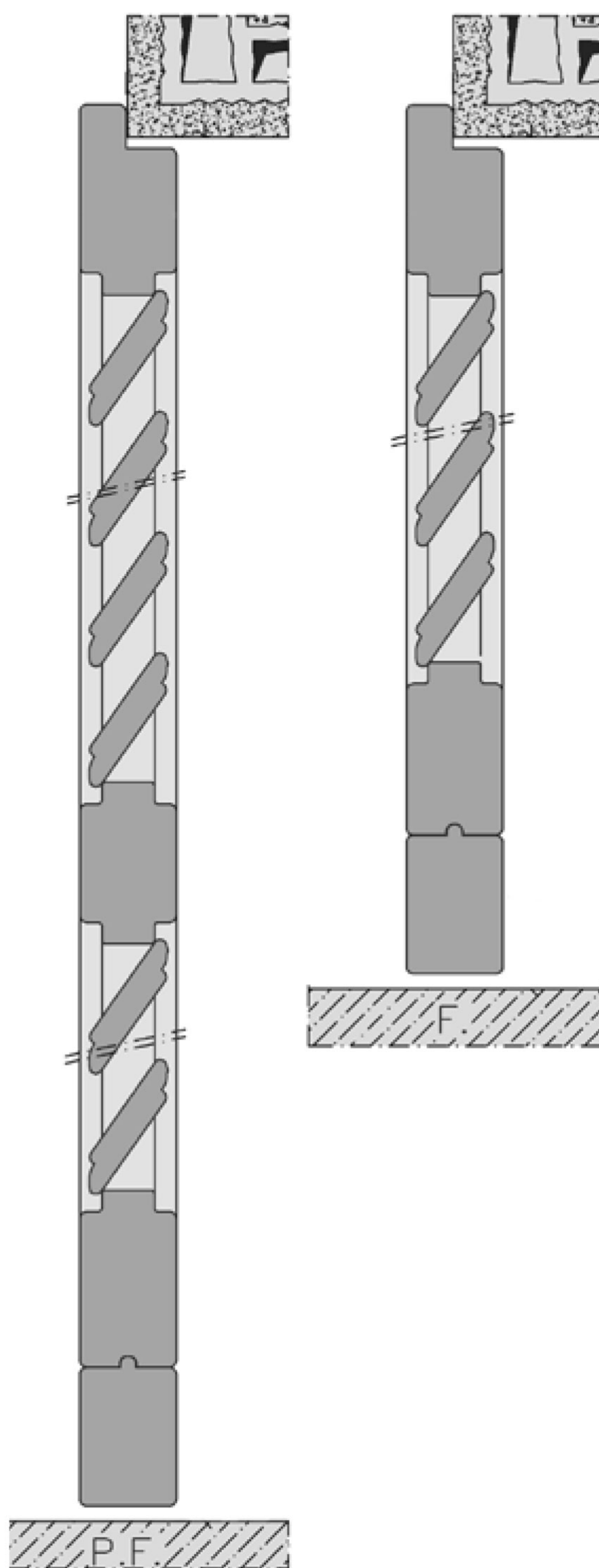
SEZIONE VERTICALE
