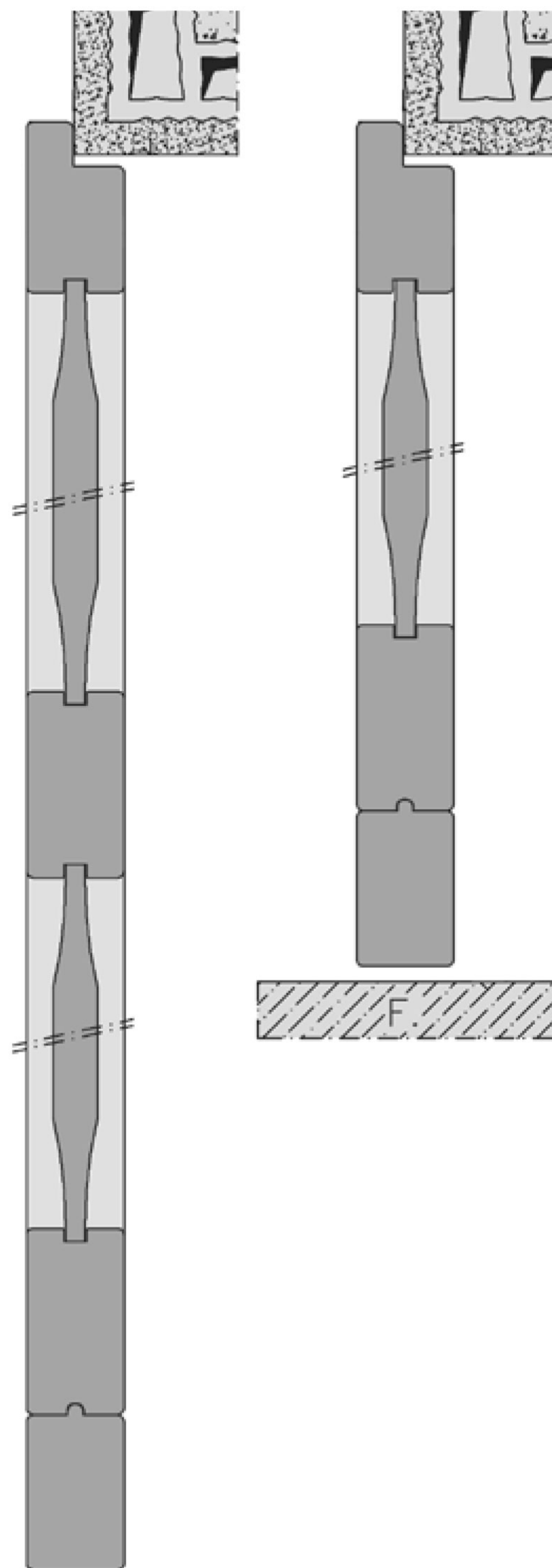
SEZIONE VERTICALE
