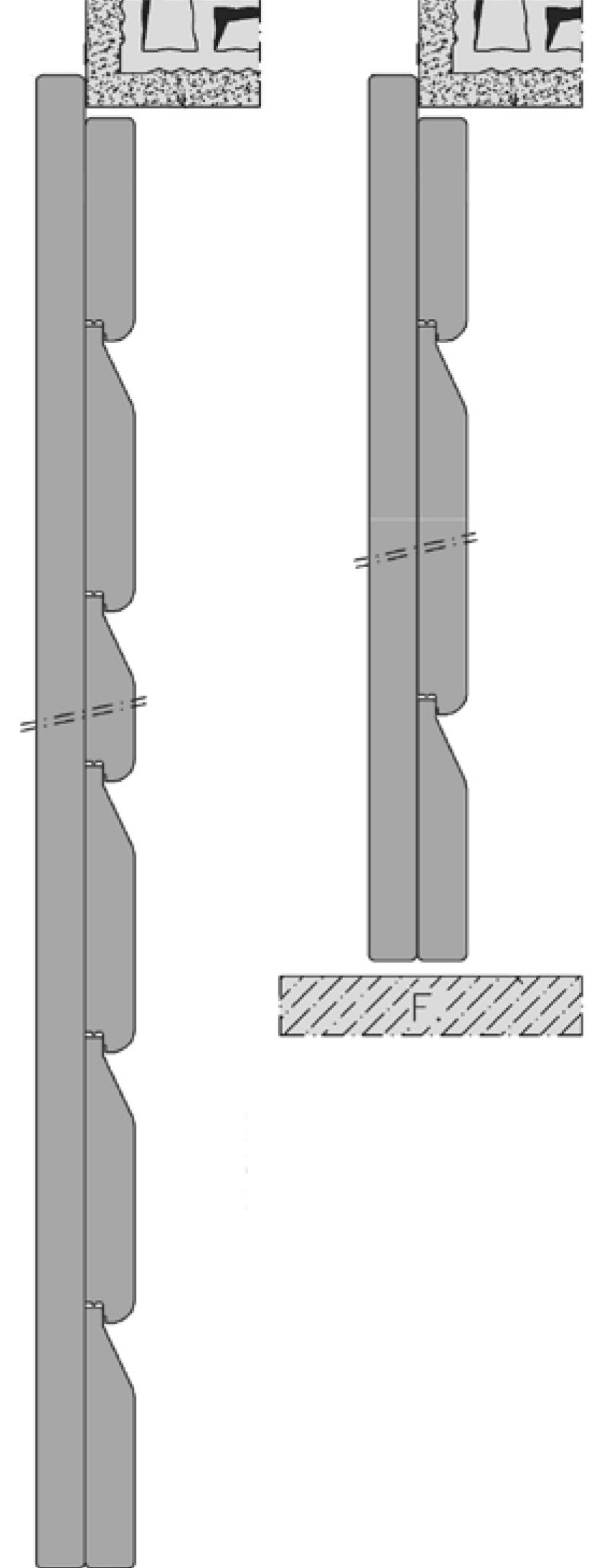
SEZIONE VERTICALE
